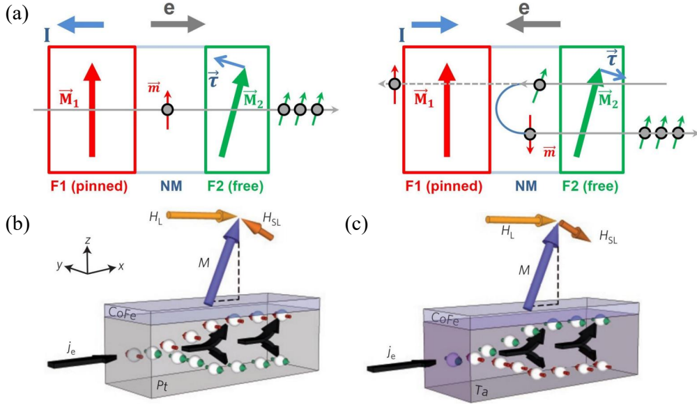
图 2.8 STT 与 SOT 原理示意图
