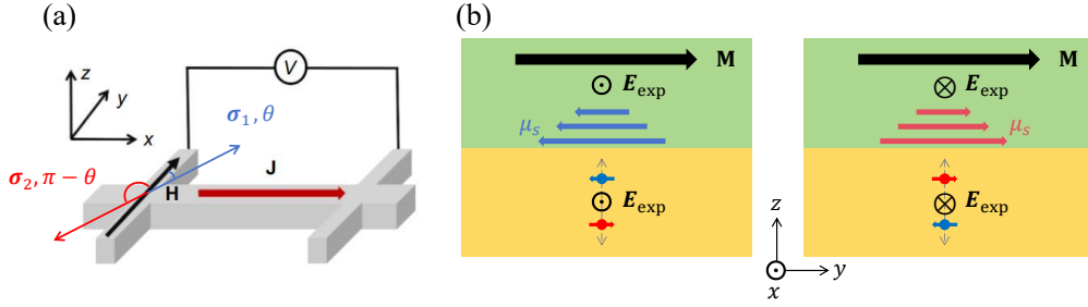
图 5.8 USMR 测量原理示意图
